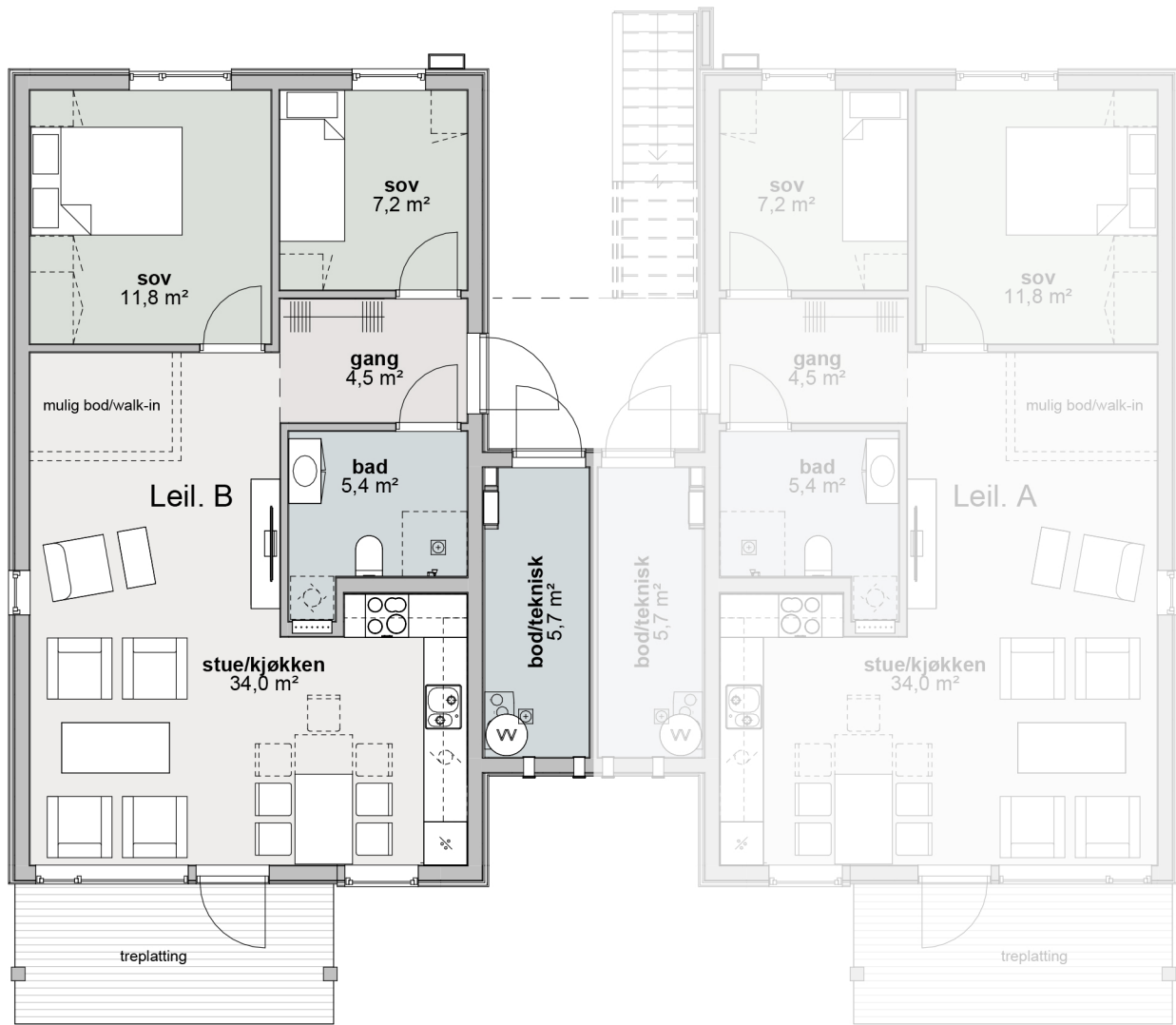
1. Etasje salgsplan 1 : 100
