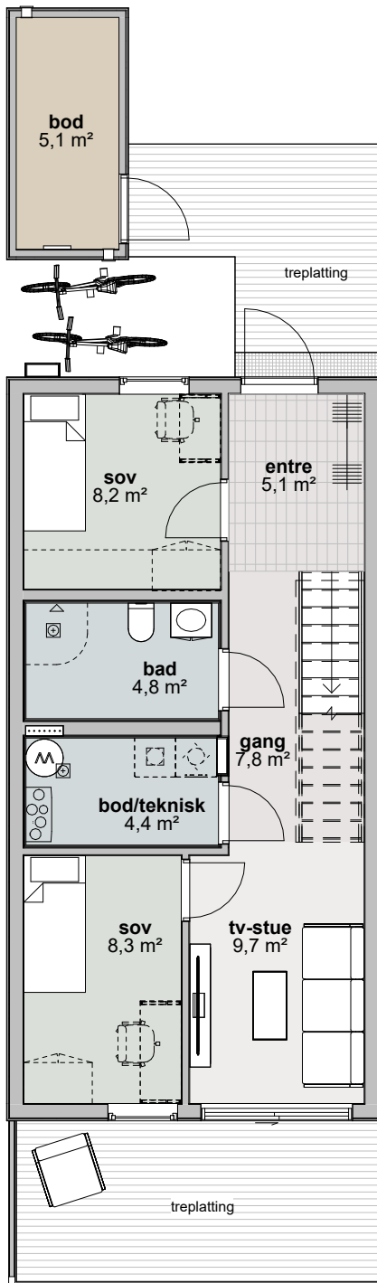
1. Etasje salgsplan 1 : 100
