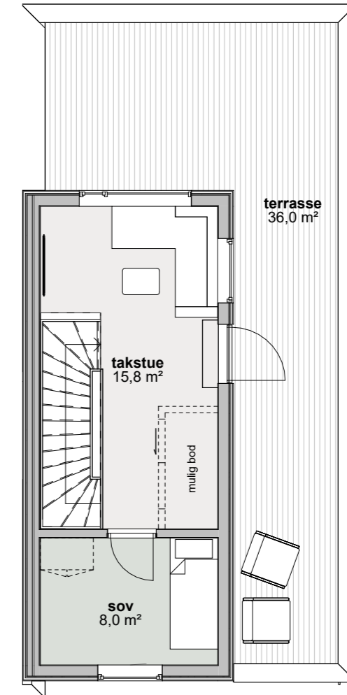
3. Etasje salgsplan C speilvendt 1 : 100
