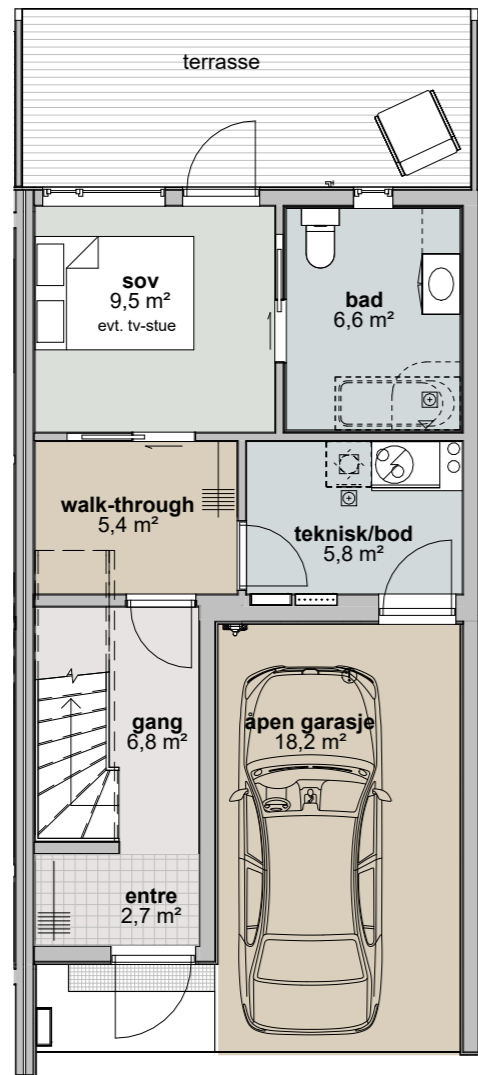
1. Etasje salgsplan C speilvendt 1 : 100
