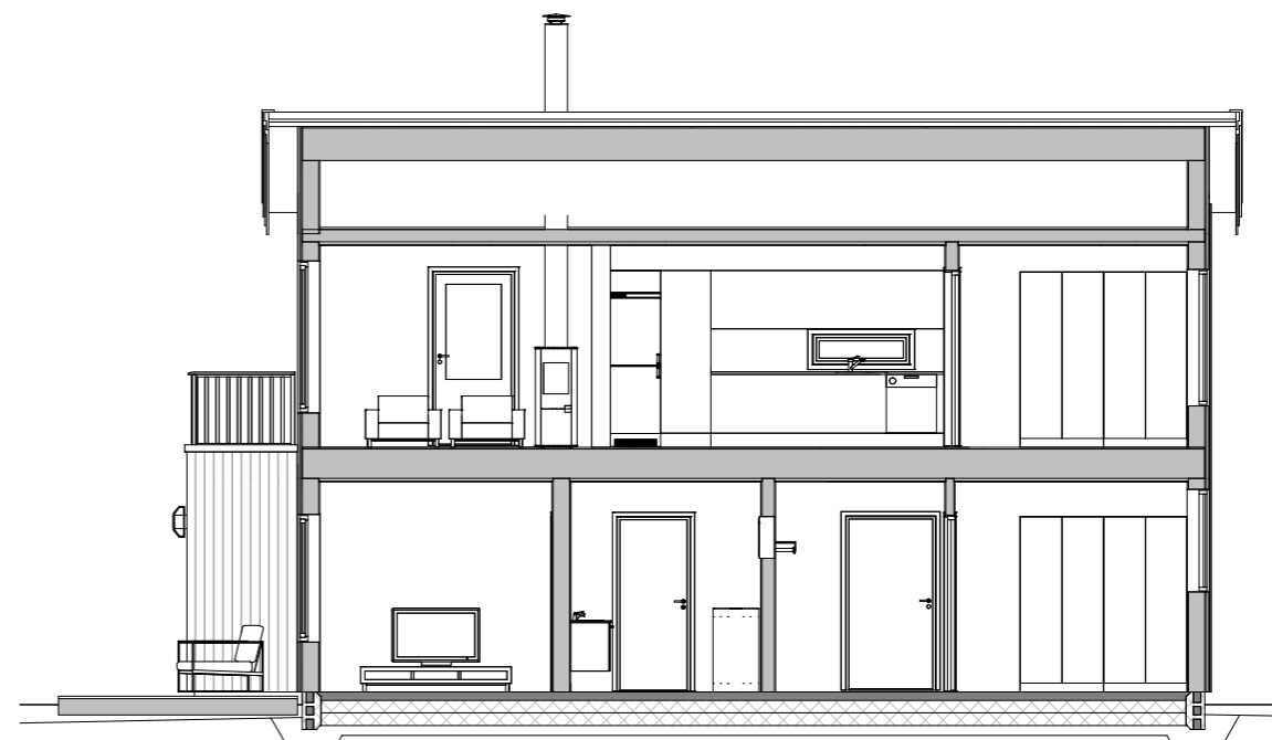
C1 1 : 100
