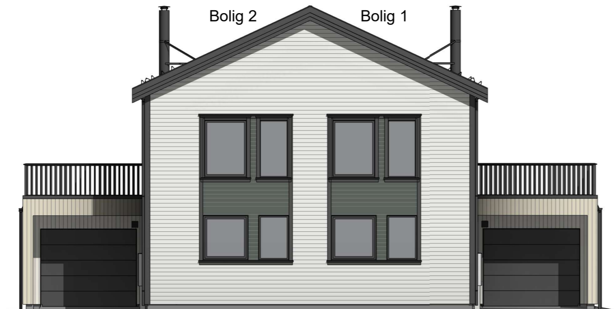
Nord 1 : 100
