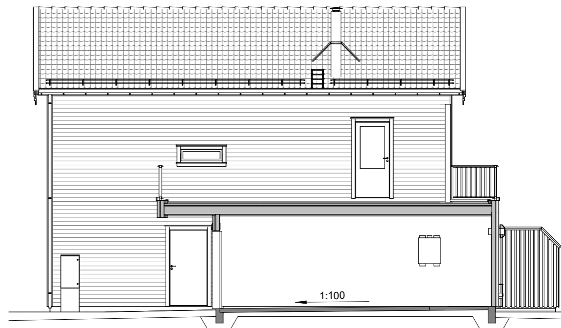
B1 1 : 100
