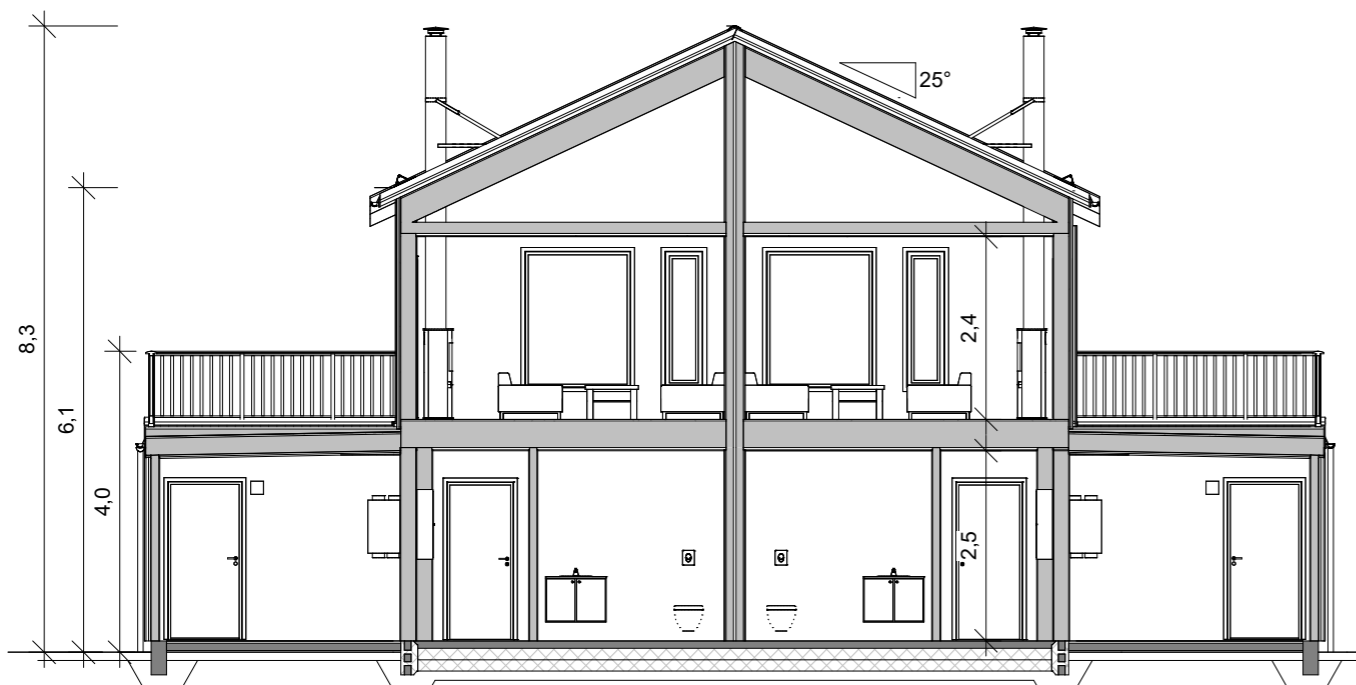
A1 1 : 100
