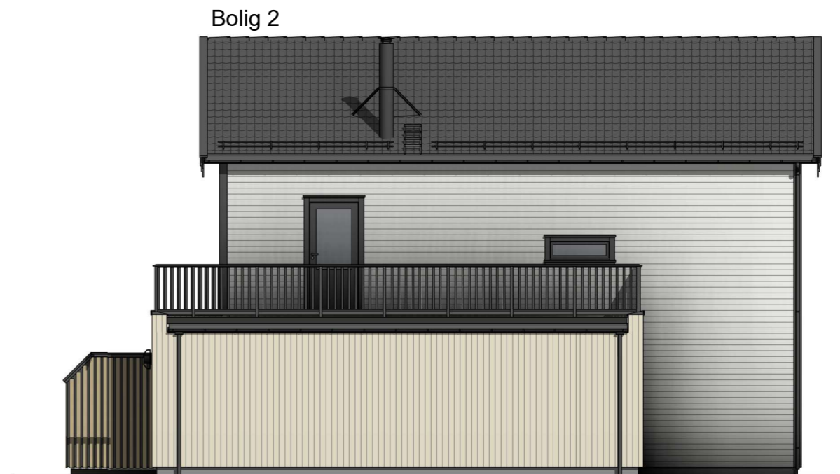
Vest 1 : 100
